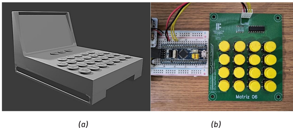
Figura 1 – (a) Modelo 3D da carenagem e (b) Protótipo do STM32 com teclado matricial.
